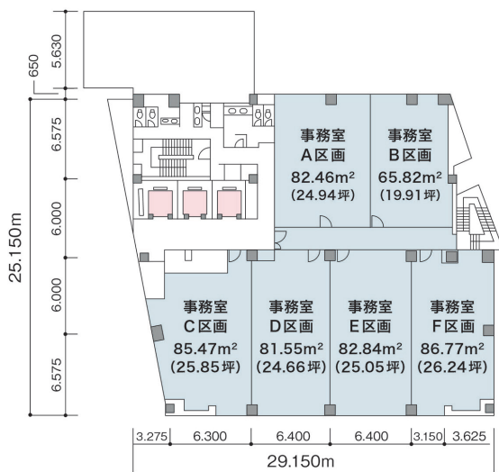
[11~12F] 平面図
