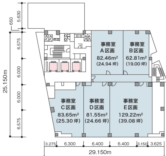
[2F] 平面図
