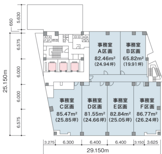
[11~12F] 平面図
