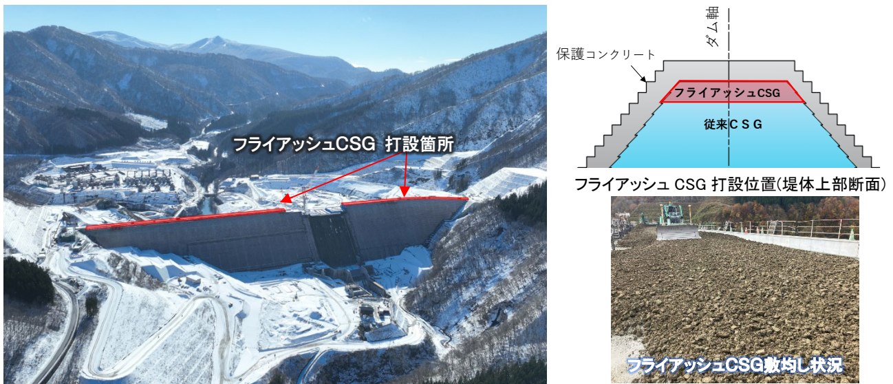
成瀬ダム堤体の一部に導入したフライアッシュ CSG
