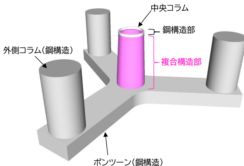
複合(ハイブリッド)構造適用箇所
