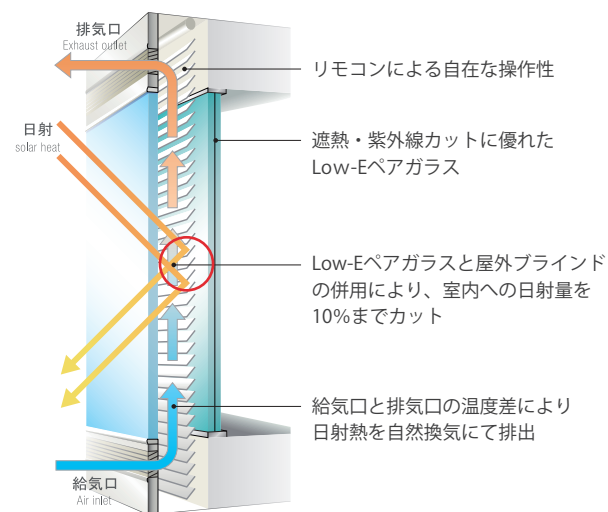
ダブルスキンカーテンウォール断面イメージ
